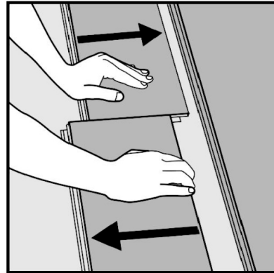
Fig12. Skil plankerne ad ved at glide vandret. Fold ikke sammen! Løft op vil beskadige endeprofiler.
