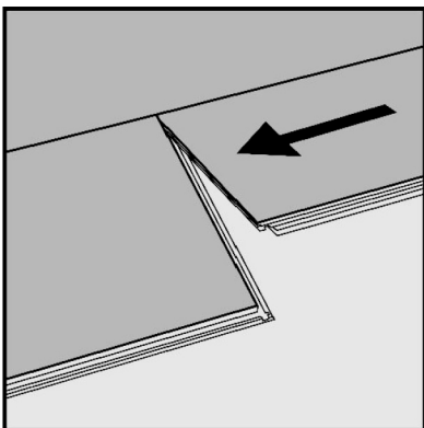
Fig8a Anden planke, anden række. Placer planken forsigtigt og stram til den korte ende af den forrige planke. Som Fig3.
